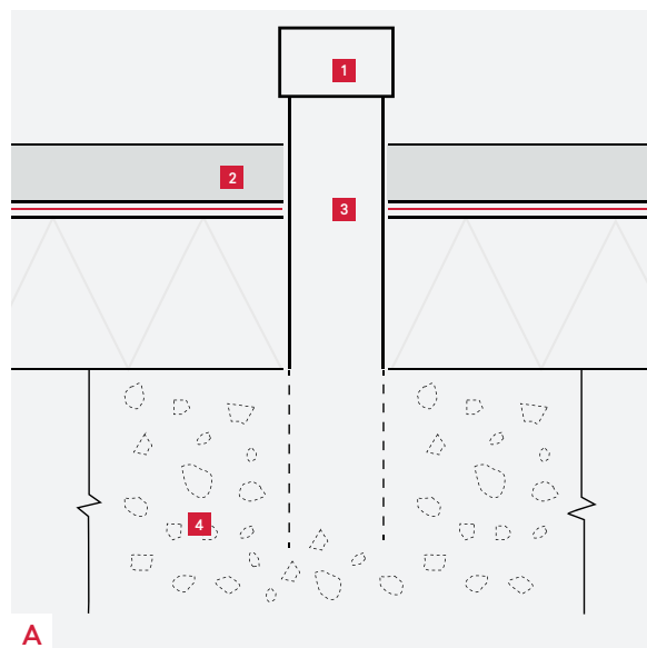
Placering af brønd
