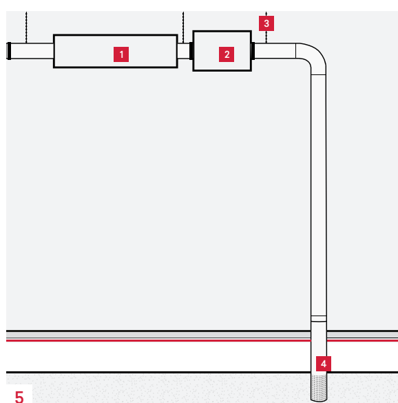
Tilslutning til ventilation
