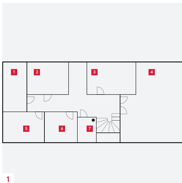
Eksempel på placering af radonbrønd i bryggers
