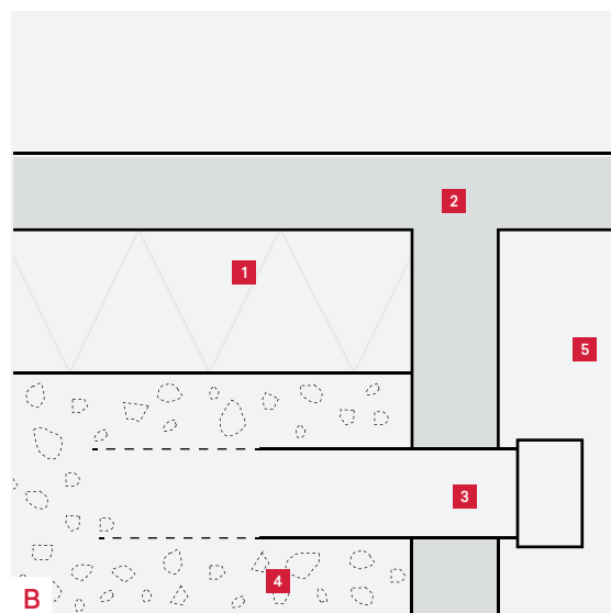
Vandret montering under plade på jord
