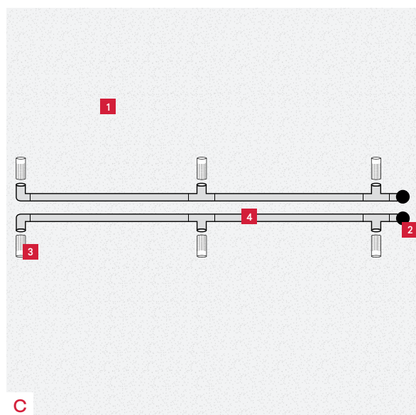
Montering af Radon Sugbrønd A400 på større områder
